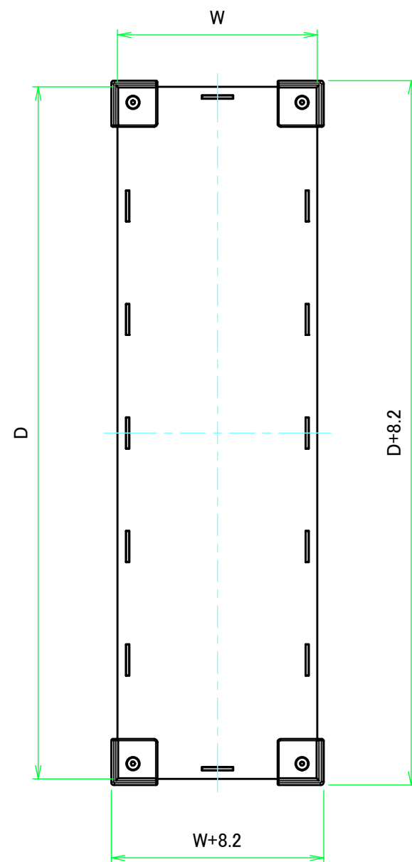
上カバー / Top cover
