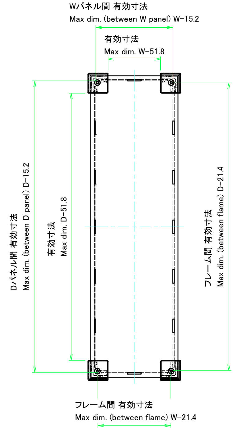
下カバー / Bottom cover
